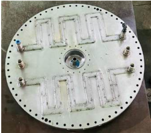
आरआरकेट हेतु एंड फ्लेंज असेम्बली
